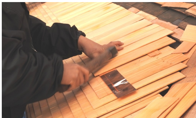
▲ 「銅板」 をこけら板の間に葺き込む様子
